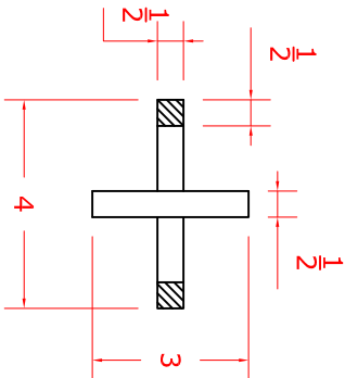
Detail 04 : Top View Scale: 3" = 1'-0"
